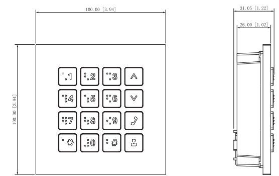
DHI-VTO4202F-MK
