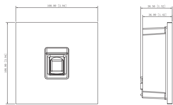
DHI-VTO4202F-MF
