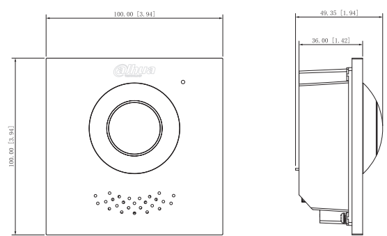
DHI-VTO4202F-P
