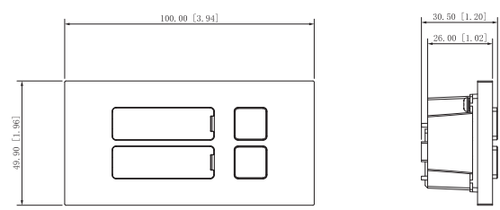
DHI-VTO4202F-MB2
